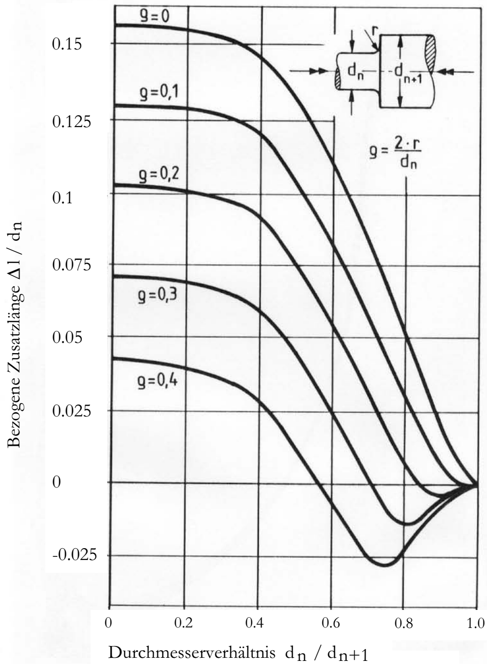
Bild 4.2-4: Bezogene Zusatzlängen für verschiedene, einfach abgesetzte Wellen mit Übergangsradius r in Abhängigkeit vom Durchmesser Verhältnis des Übergangs /4.2-3/
